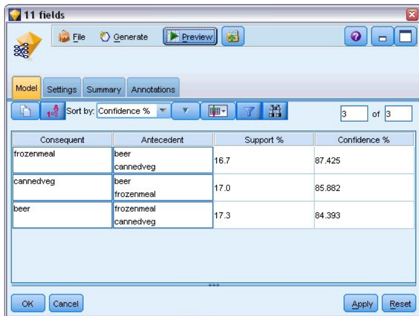
图 382. 关联规则
